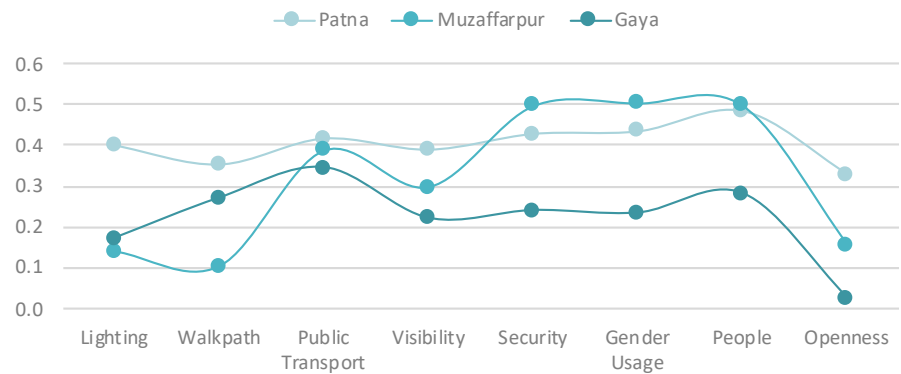
Parameter Correlation w.r.t. Feeling Parameter
